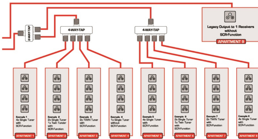
Wyjścia kaskadowe
